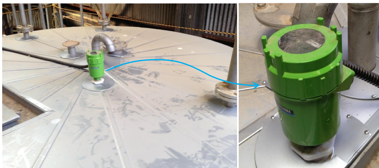
动物油脂储槽的导入事例
